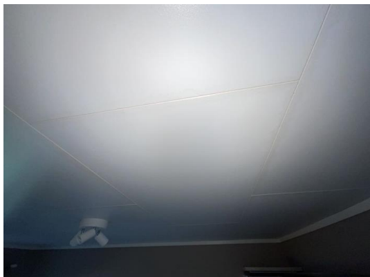
Fuktskjolder langs skjøter i himlingsplater på soverom.
