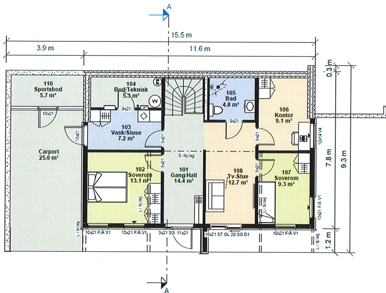
1. Etasje
