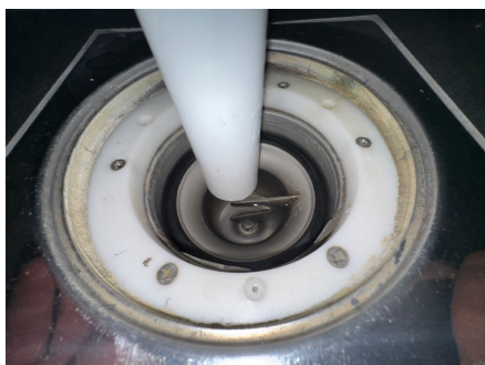
Stålsluk med klemring og synlig membran/mansjett
