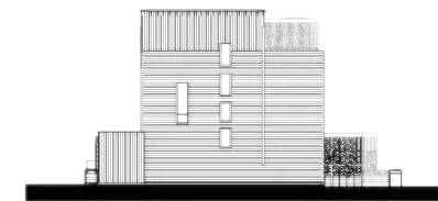
Fasade Gavl
