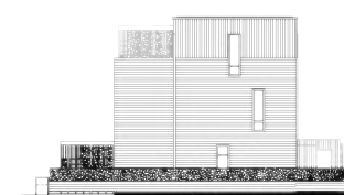
Fasade Gavl
